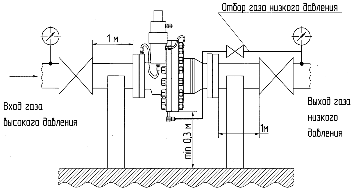
Рисунок Б2: Рекомендуемая схема установки и обвязки регулятора давления РДУ-100/50 и РДУ-100/80 редуктором-задатчиком.
