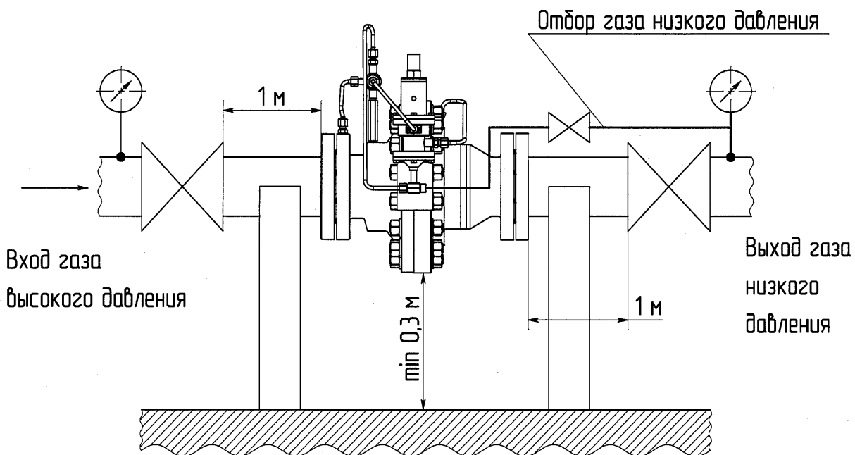
Рисунок Б3: Рекомендуемая схема установки и обвязки регулятора давления газа РДУ-64/100 и РДУ-100/100 редуктором перепада с усилителем.
