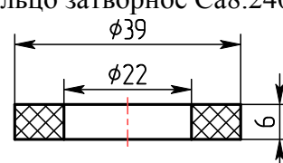
Кольцо затворное Ca8.240.062
